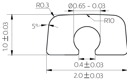
COD. 80020132 Materiale: Acciaio
