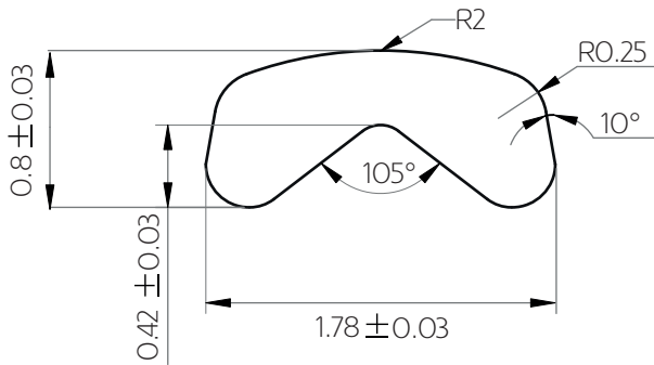
COD. 80020211 Materiale: Acciaio
