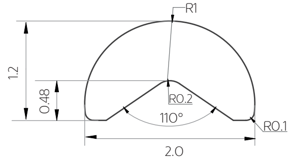
COD. 80020256 Materiale: Acciaio
