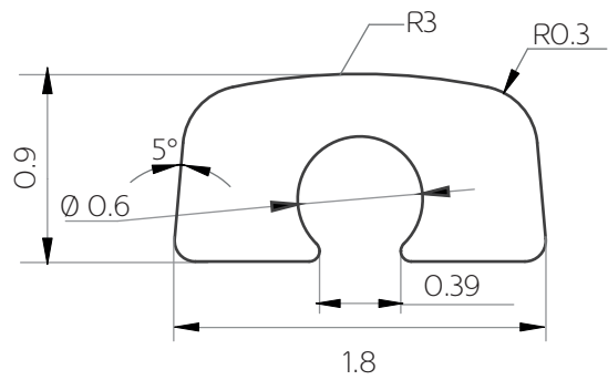
COD. 80010603 Materiale: Monel
