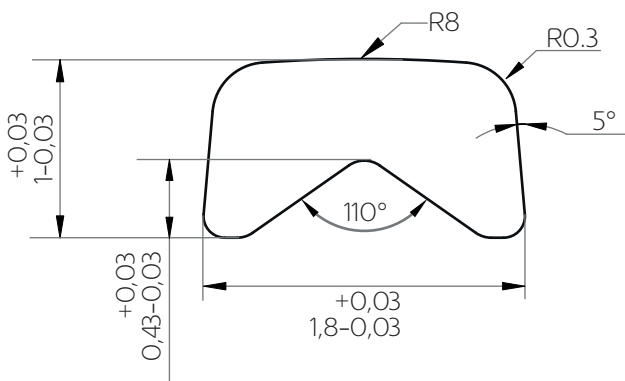
COD. 8001094 Materiale: Monel
