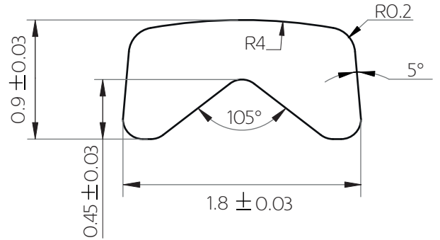
COD. 80010101 Materiale: Monel
