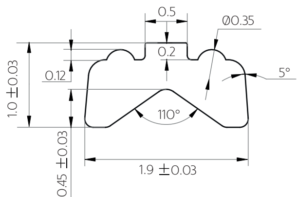
COD. 80010604 Materiale: Monel
