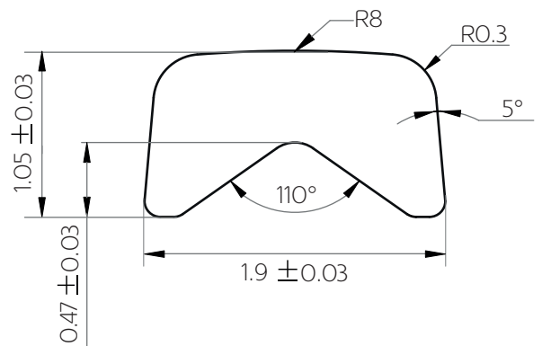
COD. 80020983 Materiale: Acciaio
