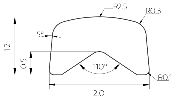
COD. 80010290 Materiale: Monel
