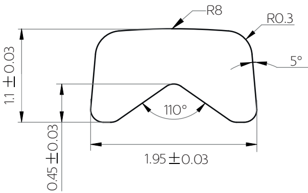
COD. 80010702 Materiale: Monel
