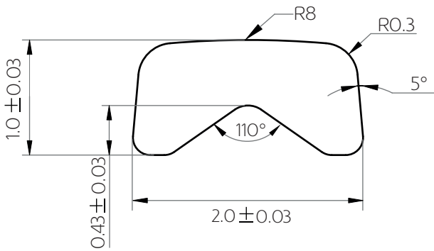
COD. 80010131 Materiale: Monel
