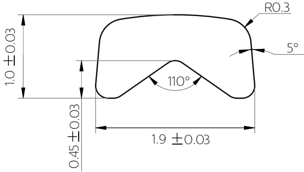
COD. 80010602 Materiale: Monel
